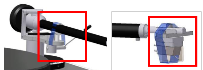
Abb. 4: Entfernen der Sicherheitsstreifen
